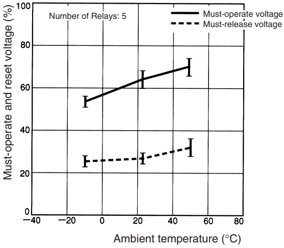
G7J 24 VDC
