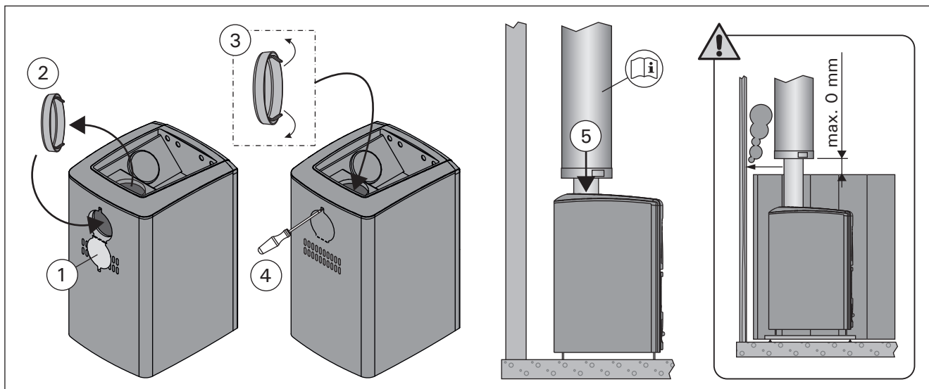
Рисунок 13. Присоединение печи к стальному дымоходу Harvia (все размеры приведены в миллиметрах) Joonis 13. Kerise ühendamine Harvia teraskorstnaga (kõik mõõtmised millimeetrites)
